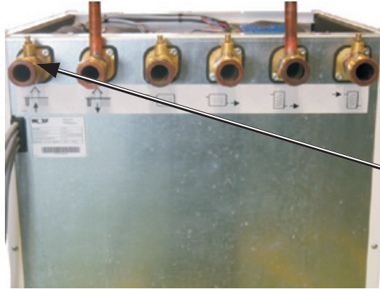
Handontluchter in de brijn-intrede
