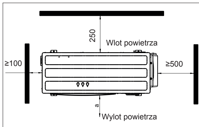
Moduł zewnętrzny widok z góry BWL-1S(B)-10/14/16
