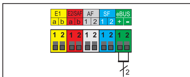
Przyłącze cyfrowych elementów sterowania (złącze eBus)
