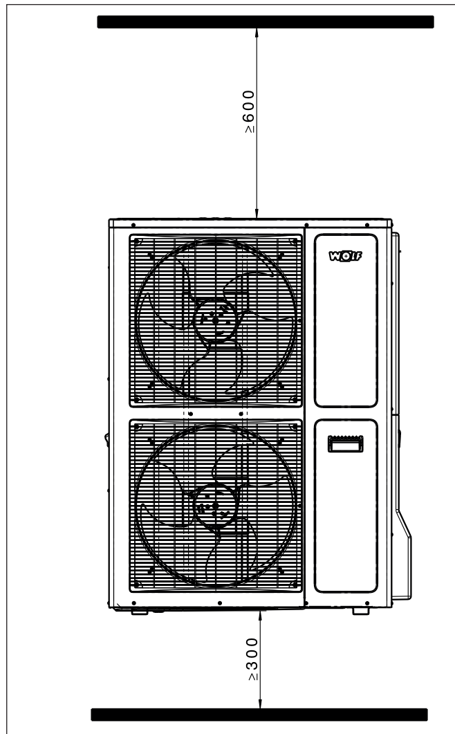
Widok z przodu, moduł zewnętrzny BWL-1S(B)-10/14/16
