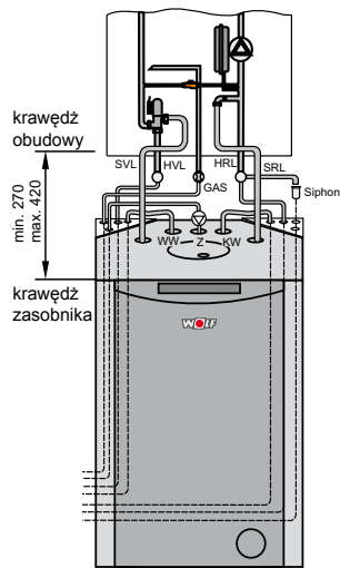
orurowanie natynkowe
