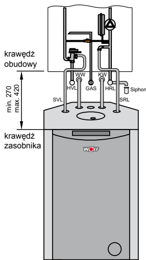
orurowanie podtynkowe
