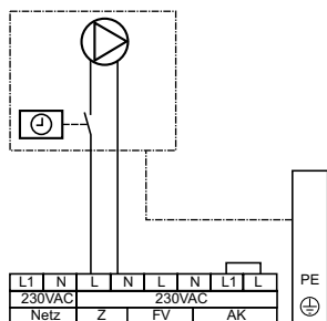
Pompa cyrkulacyjna
