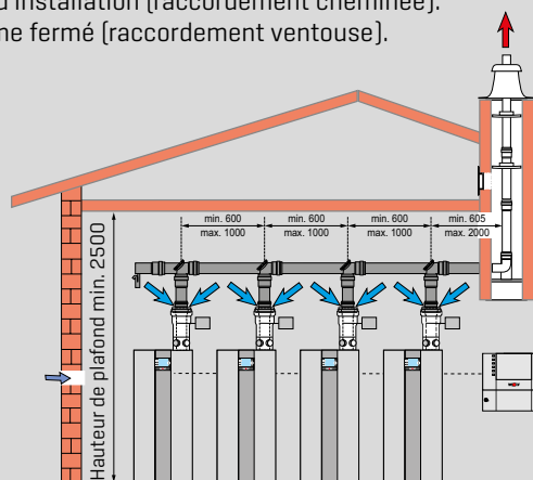
Commande en cascade avec tube de fumée collective
