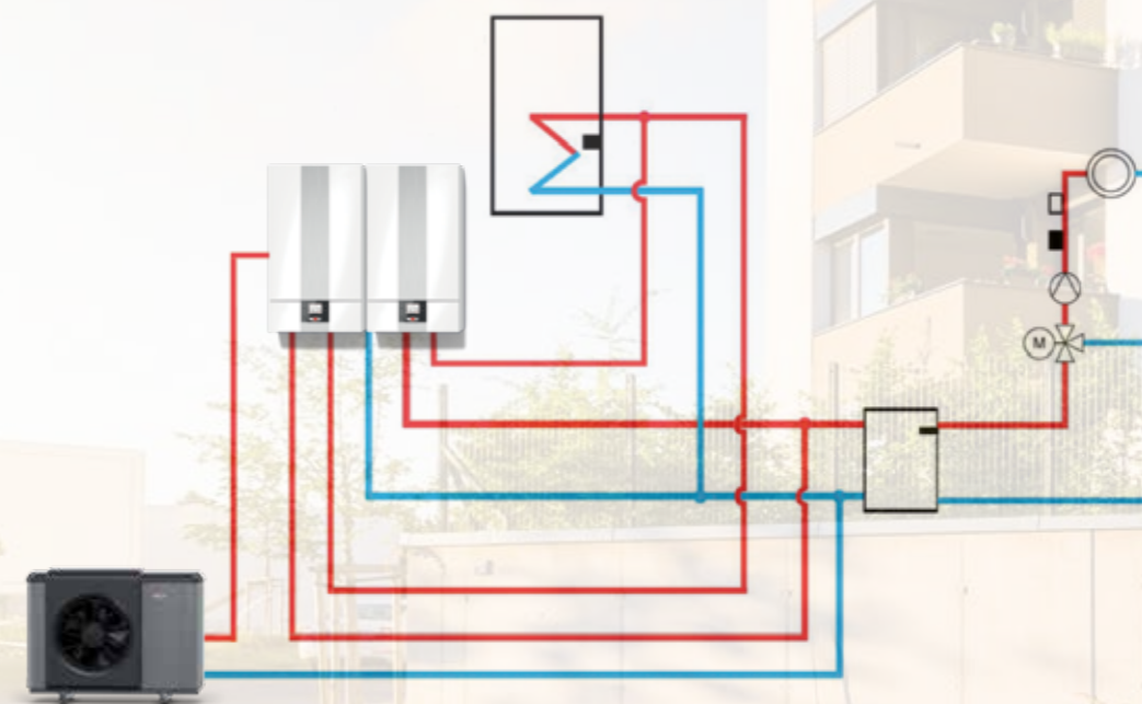
Zjednodušený príklad hydraulického schémy
