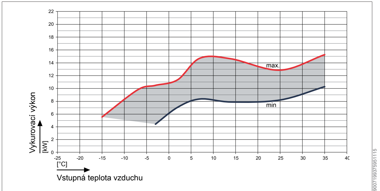
Obr. 50: Vykurovací výkon FHA-14/17 – 230 V pri teplote prívodu 55 °C
