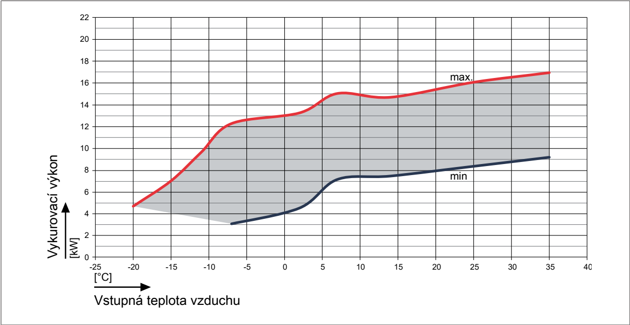
Obr. 56: Vykurovací výkon FHA-14/17 – 400 V pri teplote prívodu 45 °C
