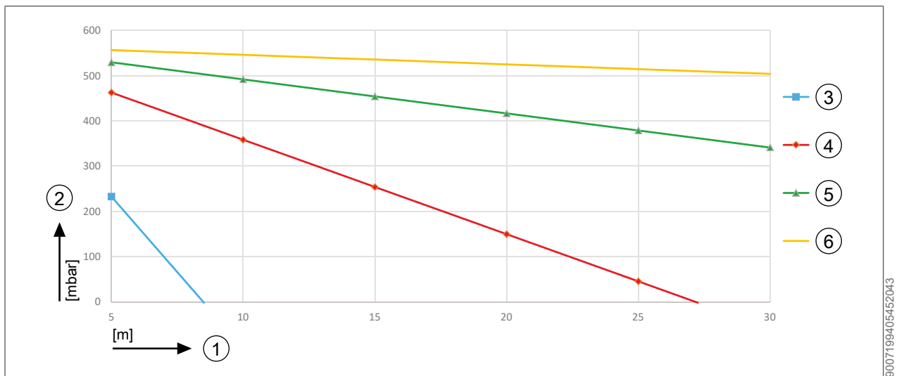
Obr. 6: FHA-14/17 Dostupná dopravná výška
