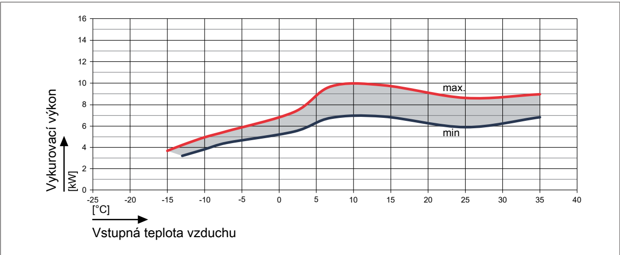
Obr. 29: Vykurovací výkon FHA-08/10 pri teplote prívodu 55 °C
