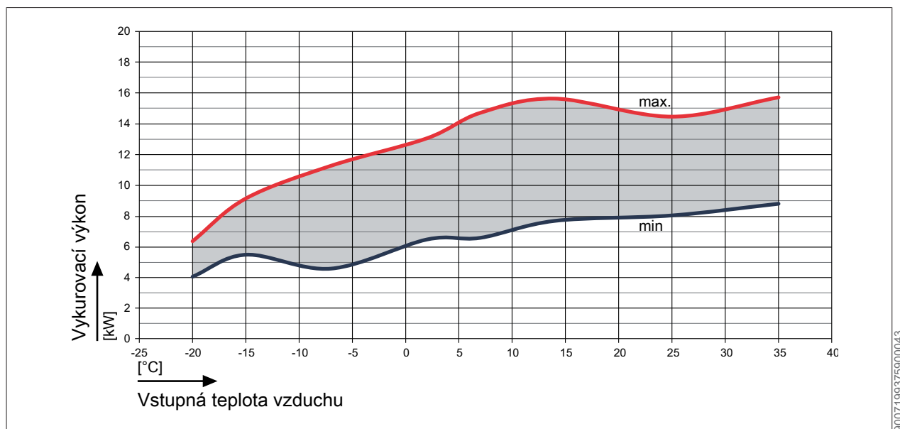
Obr. 34: Vykurovací výkon FHA-11/14 – 230 V pri teplote prívodu 35 °C
