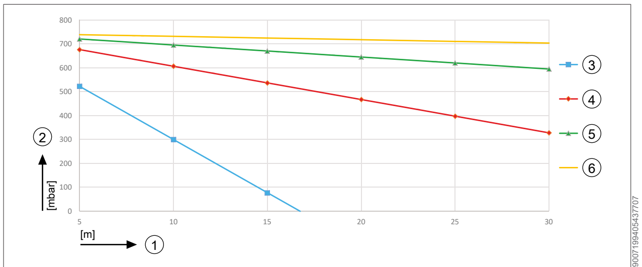
Obr. 5: FHA-11/14 Dostupná dopravná výška
