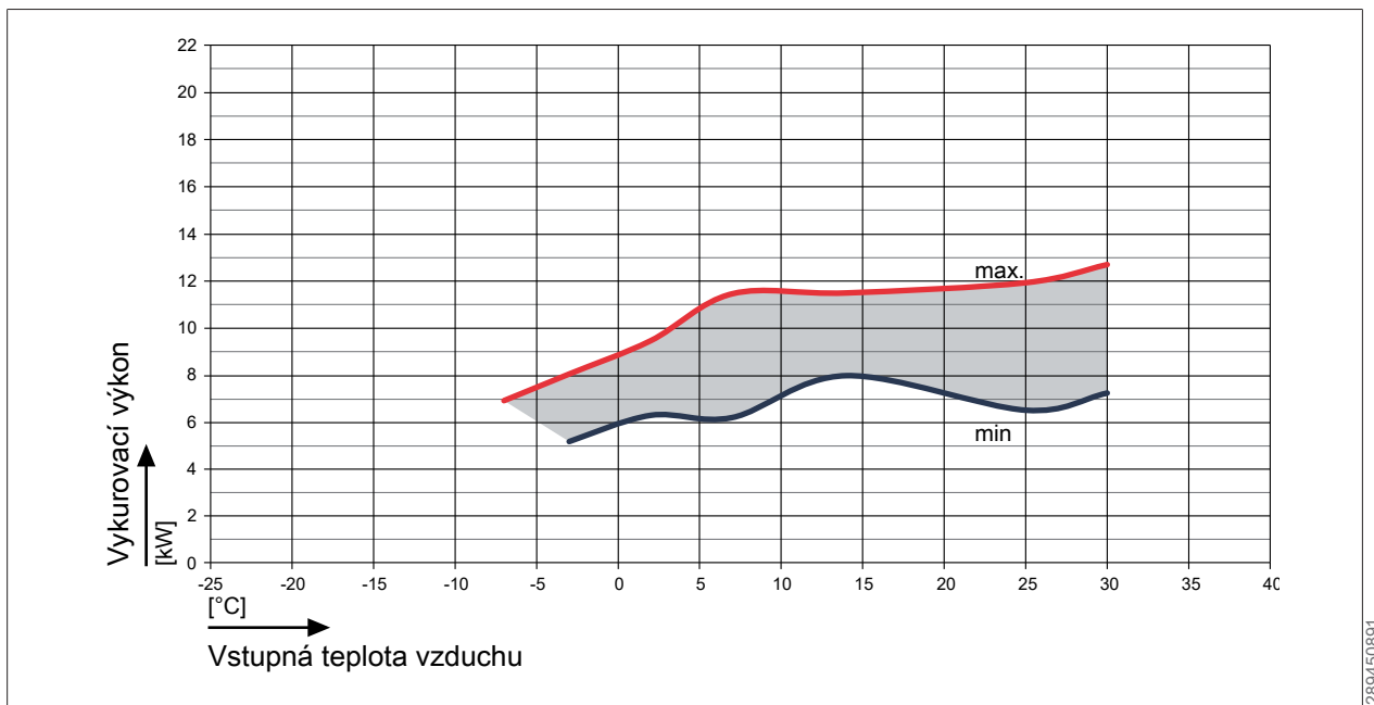
Obr. 58: Vykurovací výkon FHA-14/17 – 400 V pri teplote prívodu 60 ( \pm 2 ) °C
