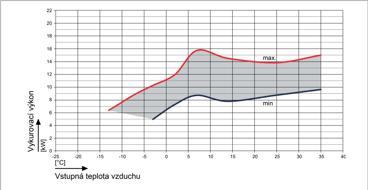
Obr. 57: Vykurovací výkon FHA-14/17 – 400 V pri teplote prívodu 55 °C
