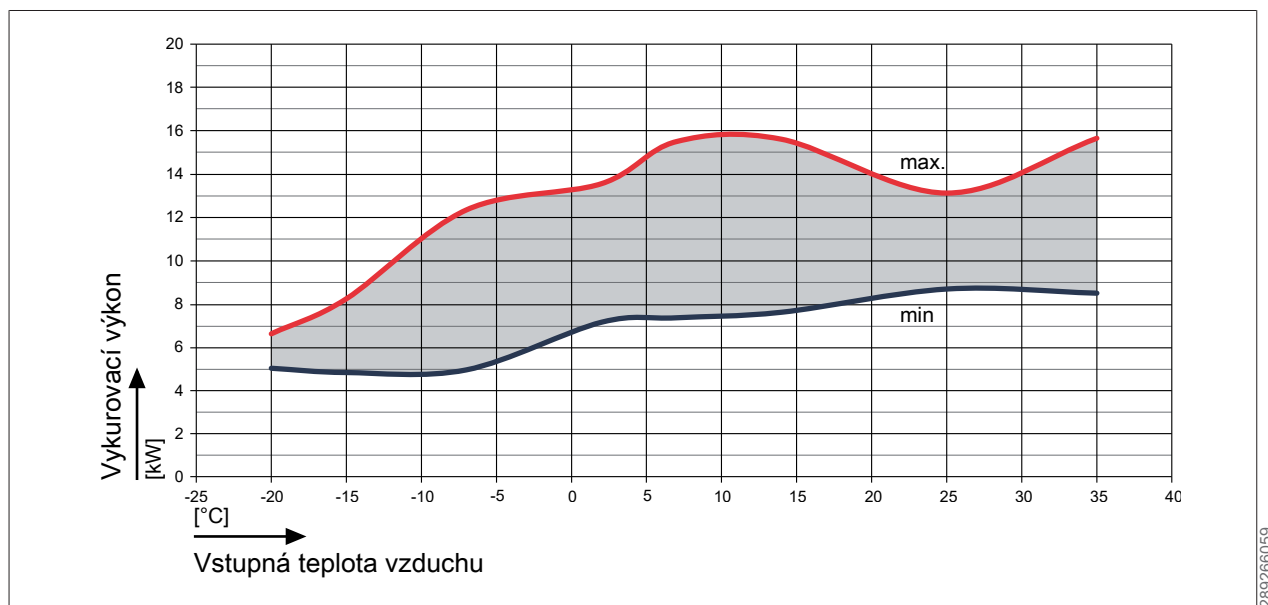
Obr. 33: Vykurovací výkon FHA-11/14 – 230 V pri teplote prívodu 25 °C
