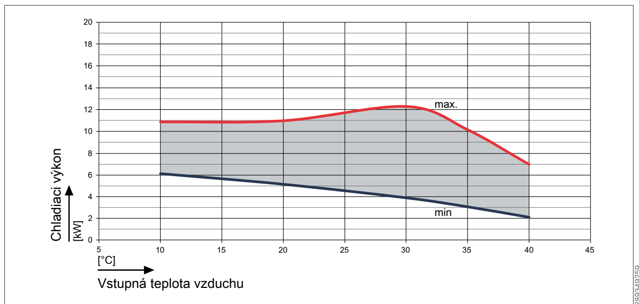
Obr. 39: Chladiaci výkon FHA-11/14 – 230 V pri teplote prívodu 7 °C
