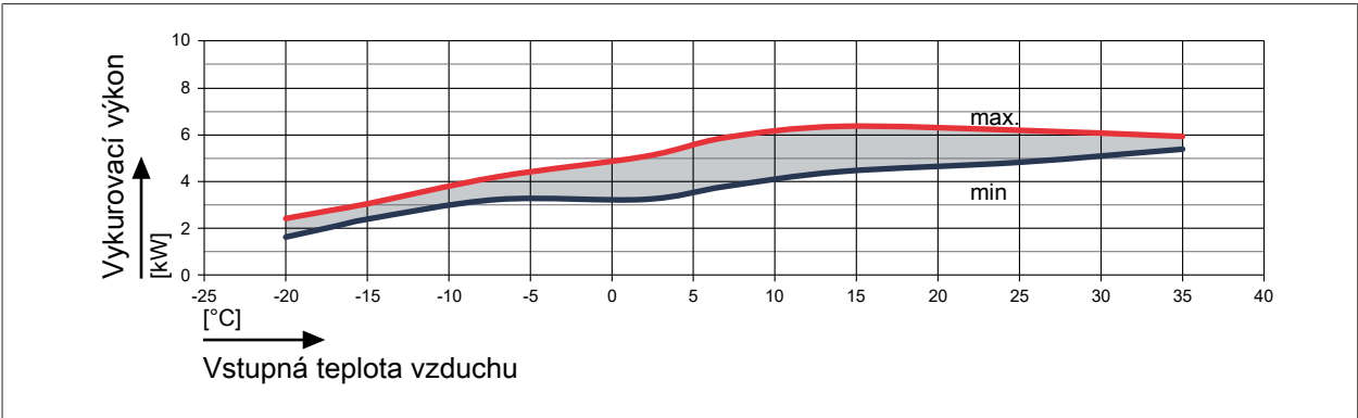
Obr. 14: Vykurovací výkon FHA-05/06 pri teplote prívodu 45 °C
