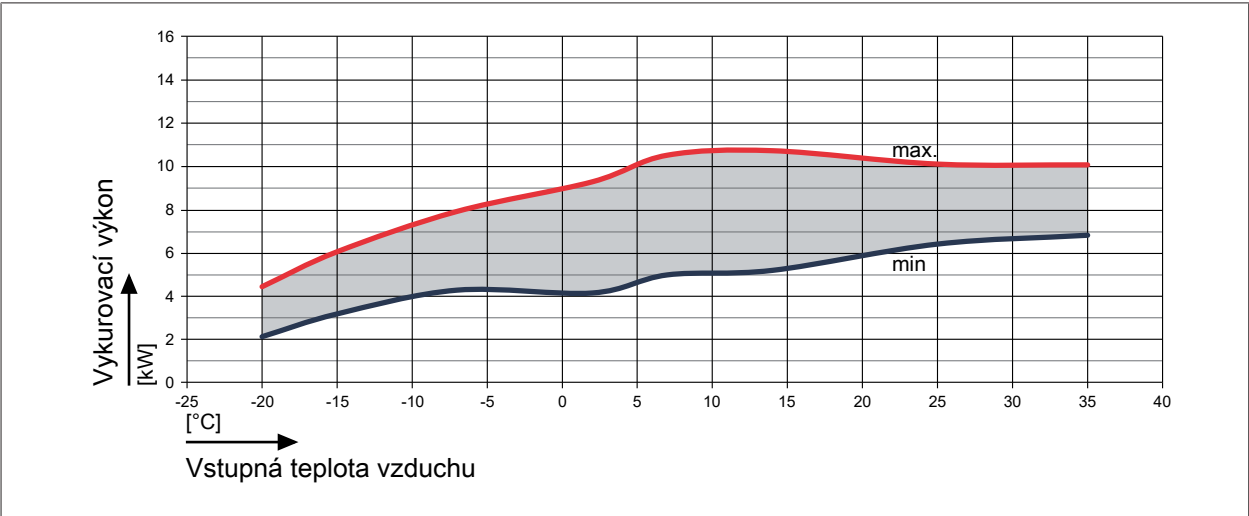
Obr. 28: Vykurovací výkon FHA-08/10 pri teplote prívodu 45 °C
