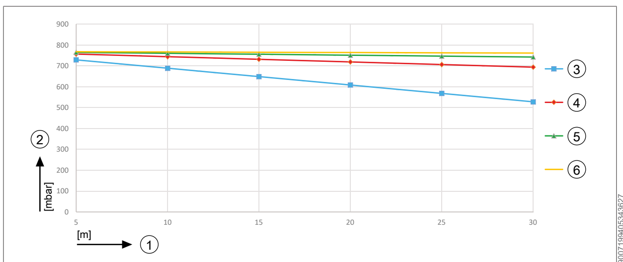
Obr. 2: FHA-05/06 Dostupná dopravná výška
