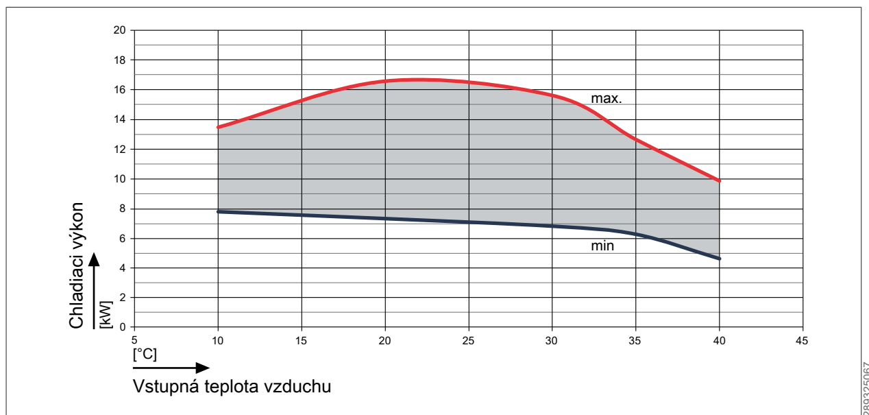
Obr. 38: Chladiaci výkon FHA-11/14 – 230 V pri teplote prívodu 18 °C
