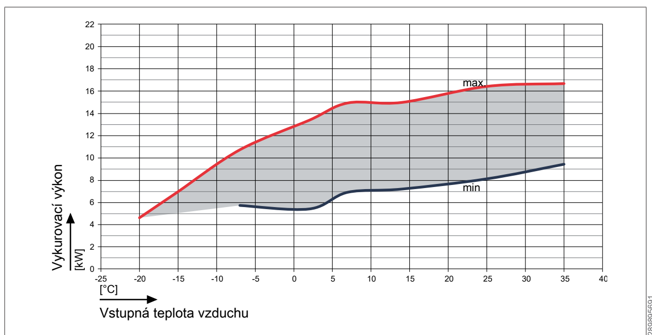
Obr. 49: Vykurovací výkon FHA-14/17 – 230 V pri teplote prívodu 45 °C
