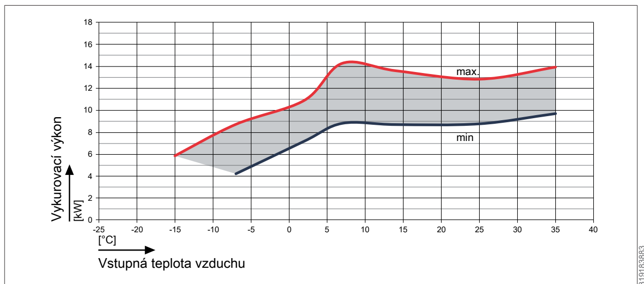
Obr. 43: Vykurovací výkon FHA-11/14 – 400 V pri teplote prívodu 55 °C
