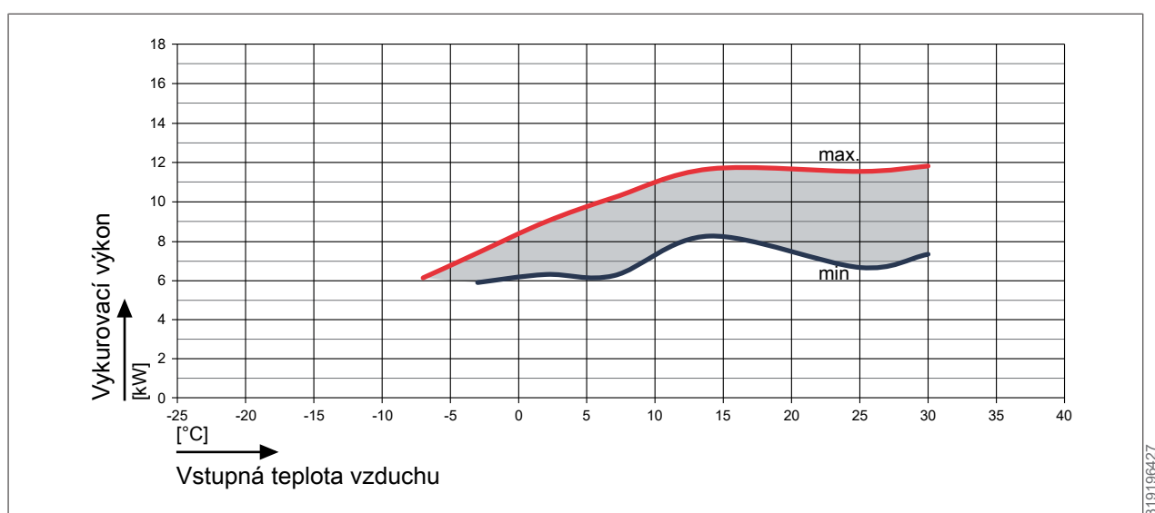
Obr. 44: Vykurovací výkon FHA-11/14 – 400 V pri teplote prívodu 60 (± 2) °C
