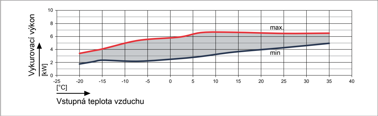
Obr. 12: Vykurovací výkon FHA-05/06 pri teplote prívodu 25 °C
