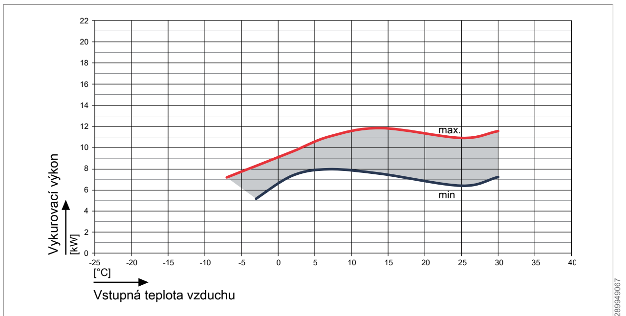
Obr. 51: Vykurovací výkon FHA-14/17 – 230 V pri teplote prívodu 60 (± 2) °C
