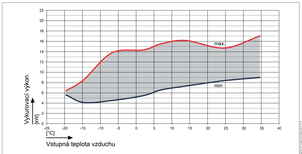
Obr. 48: Vykurovací výkon FHA-14/17 – 230 V pri teplote prívodu 35 °C
