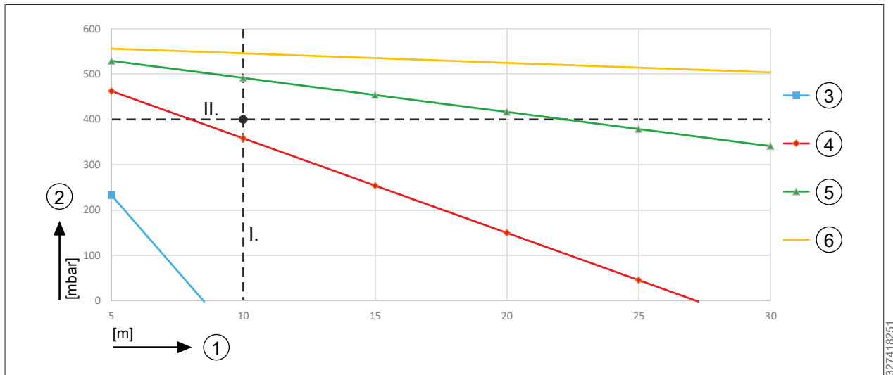
Obr. 1: FHA-14/17 Dostupná dopravná výška
