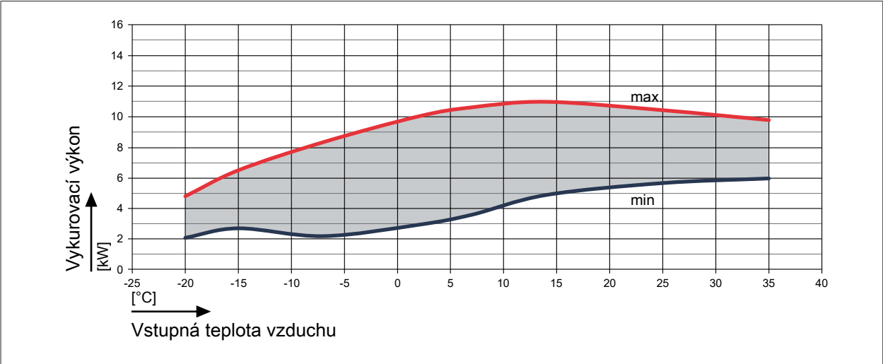
Obr. 27: Vykurovací výkon FHA-08/10 pri teplote prívodu 35 °C
