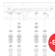
Přípoj. sada armatur pro hydr. připojení nad i pod omítku
