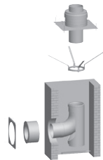
Souprava do šachty 200/200
