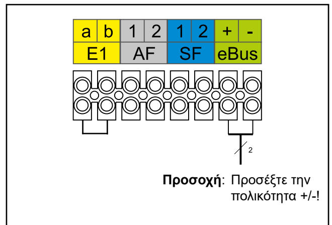
Εικόνα: Σύνδεση ψηφιακού εξαρτήματος ρυθμίσεων Wolf (θύρα επικοινωνίας eBus)
