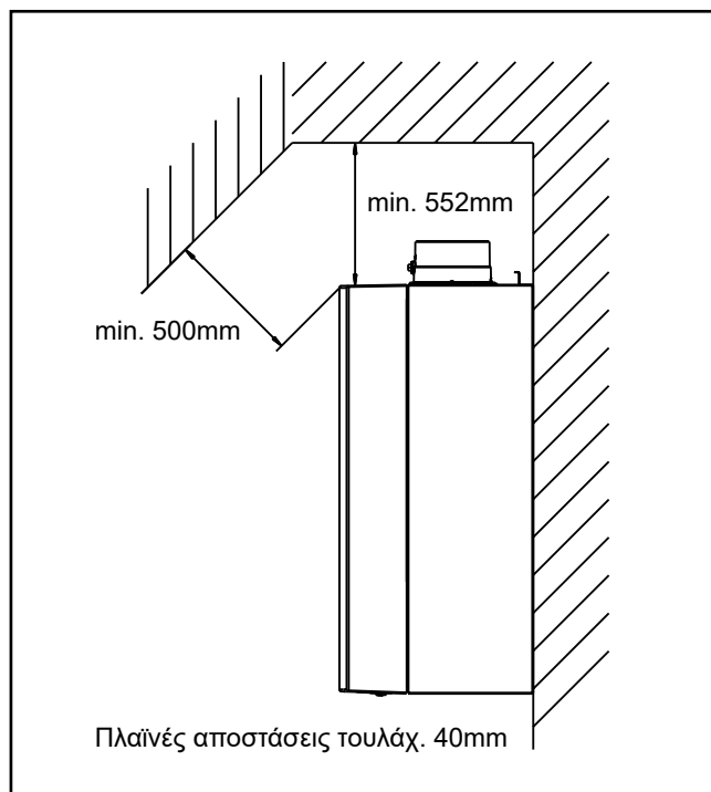
Εικόνα: Ελάχιστες αποστάσεις
