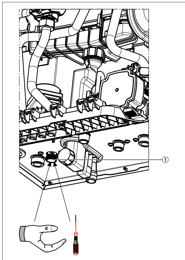
Εικόνα: Διάταξη πλήρωσης ενσωματωμένη στη συσκευή κατά την παράδοση
