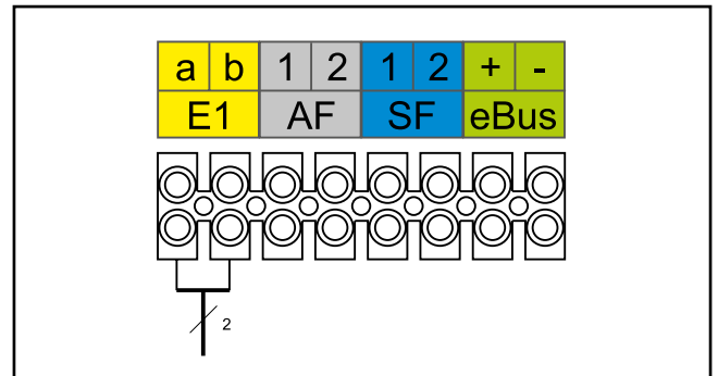
Εικόνα: Σύνδεση εισόδου E1
