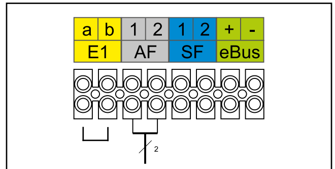
Εικόνα: Σύνδεση εξωτερικού αισθητήρα
