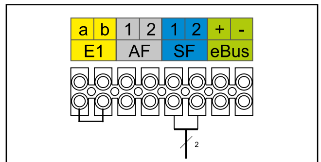
Εικόνα: Σύνδεση αισθητήρα μπόιλερ
