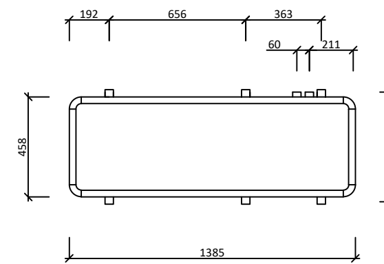
PŮDORYS:
