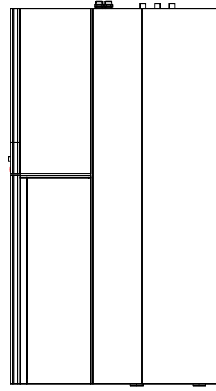
BOKORYS ( PRAVÝ )
