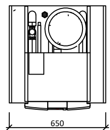
PŮDORYS
