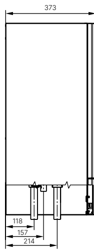
Vnútorná jednotka Bočný pohľad
