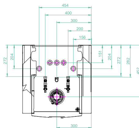
POHLED SHORA
