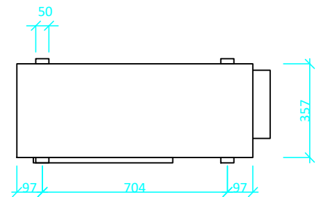
Vnější jednotka BWL-1S(B)-05/07
