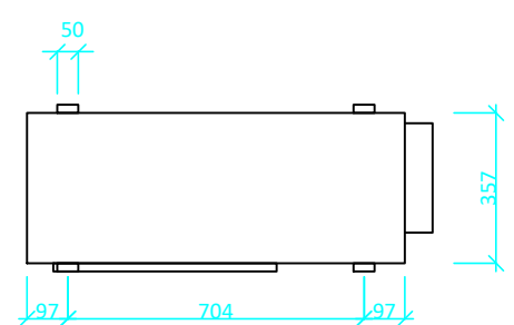
Vnější jednotka BWL-1S(B)-10/14/16
