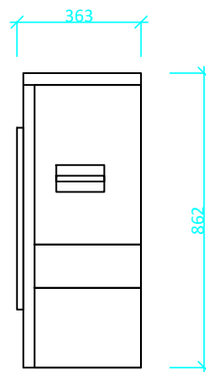
Vnější jednotka BWL-1S(B)-05/07
