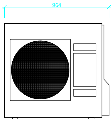
Vnější jednotka BWL-1S(B)-05/07
