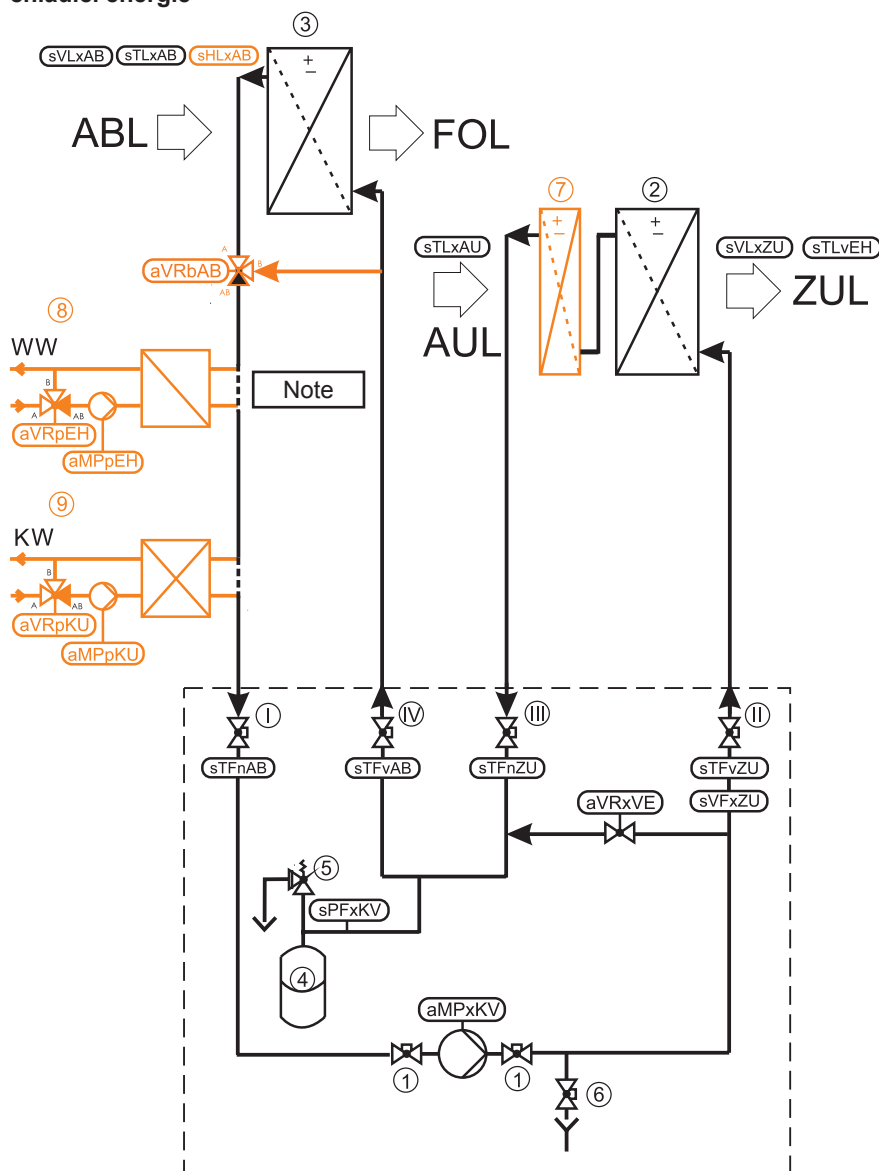
funkční schéma hydraulické jednotky s dodáváním energie
