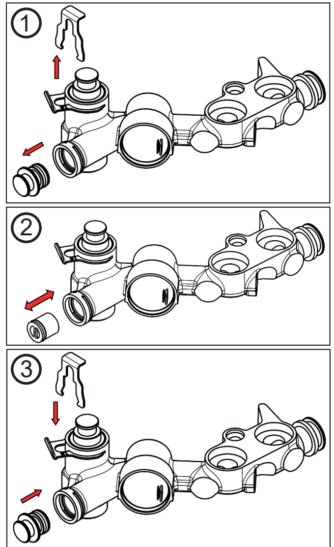
Εικόνα: Αντικατάσταση περιοριστή ροής
