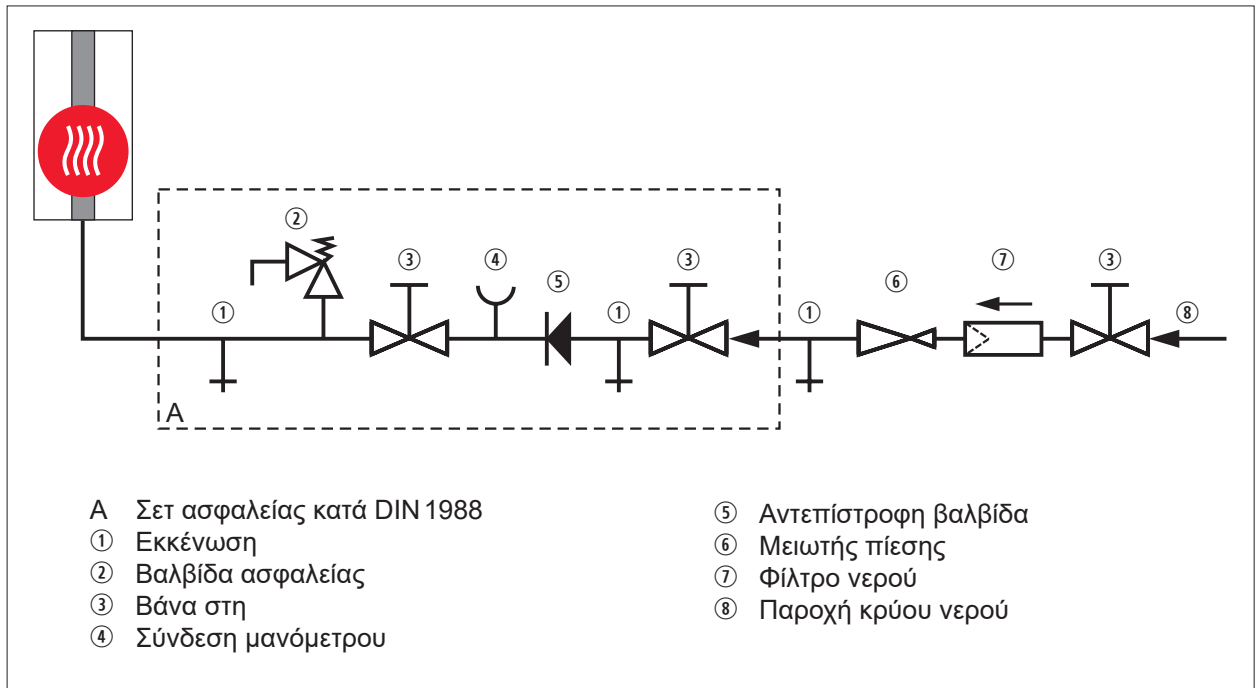
Εικόνα: Σύνδεση κρύου νερού κατά DIN 1988
