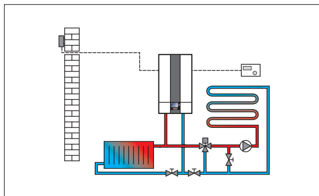
Εικόνα: Ενδοδαπέδια θέρμανση (παράδειγμα)
