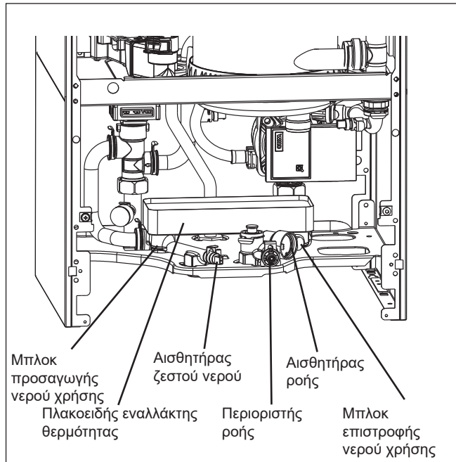
Εικόνα: Σωληνώσεις συσκευής συνδυασμένης λειτουργίας
