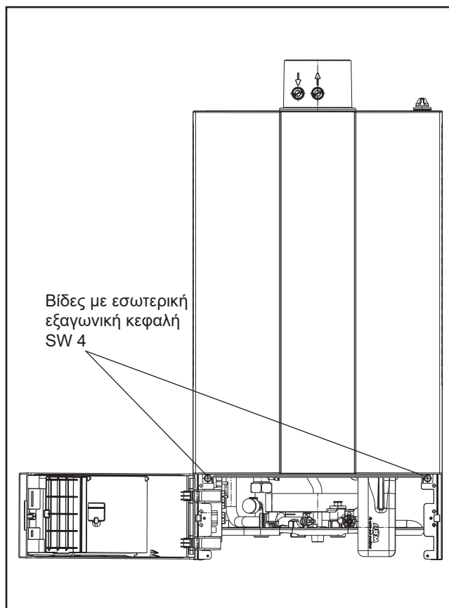
Εικόνα: Πρόσοψη, καπάκι πίνακα ρυθμίσεων πλήρως ανοιχτό
