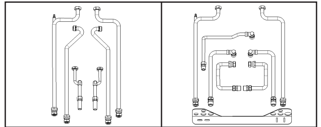
Εικόνα: Σετ σύνδεσης για μπόιλερ WOLF CSW-120 Εγκατάσταση κάτω από τον σοβά (εξάρτημα)
