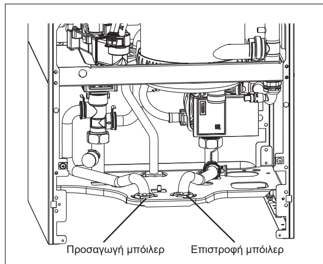
Εικόνα: Μπλοκ σύνδεσης αποσυναρμολογημένο
