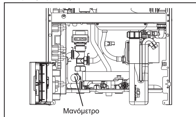
Εικόνα: Μανόμετρο
