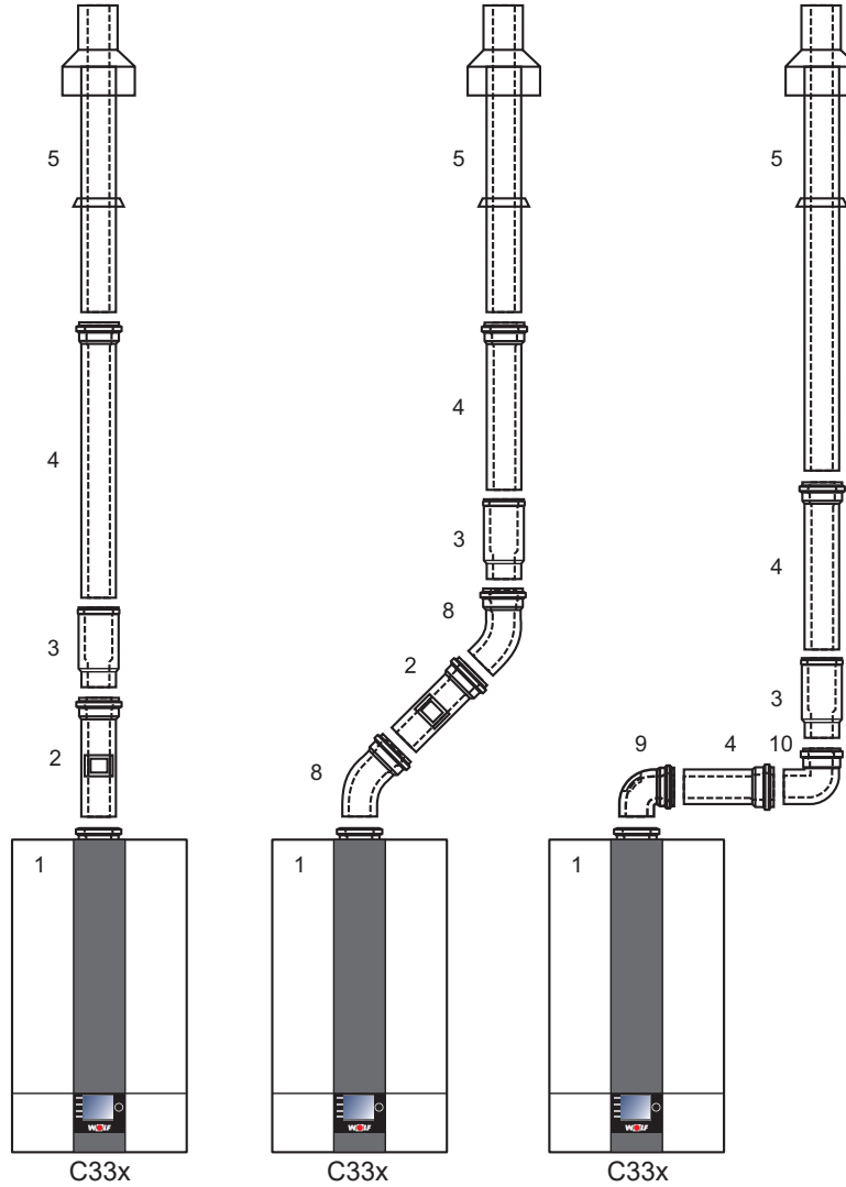
Παραδείγματα δυνατοτήτων συνδέσεων κλειστού θαλάμου (κάθετα)
