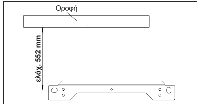
Εικόνα: Οπές για γωνία ανάρτησης
