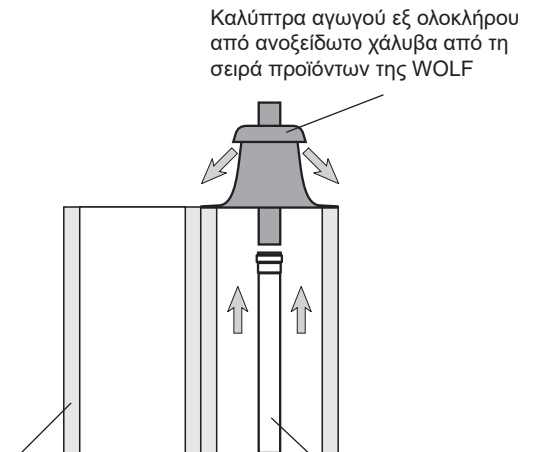
Καπνοδόχος T400
