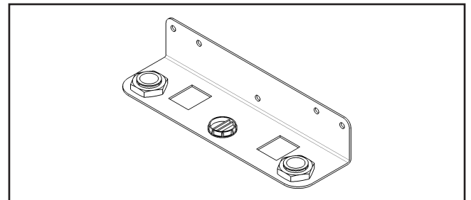
Εικόνα: Βραχίονας σύνδεσης για την έκδοση πάνω από τον σοβά (εξάρτημα) για CGB-2
