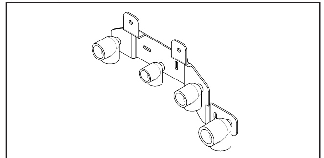
Εικόνα: Κονσόλα περιβλήματος για κάτω από τον σοβά (εξάρτημα) για CGB-2
