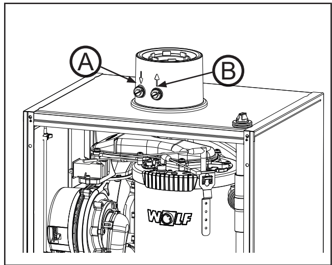
Εικόνα: Μέτρηση αέρα αναρρόφησης και παραμέτρων απαερίων
