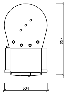
PŮDORYS
