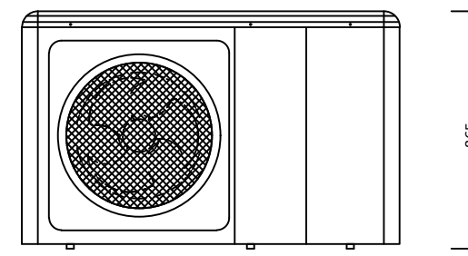
ČELNÍ POHLED:
