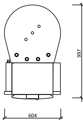
PŮDORYS
