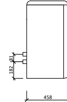
BOKORYS ( LEVÝ ) :
