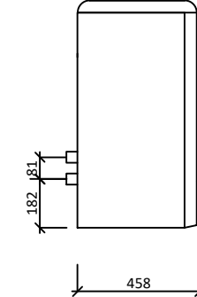
BOKORYS ( LEVÝ ) :
