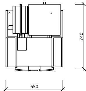
PŮDORYS
