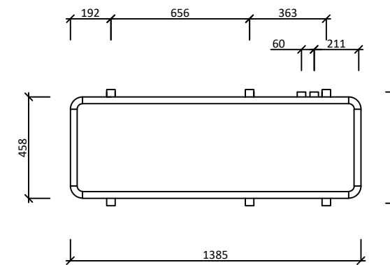
PŮDORYS:
